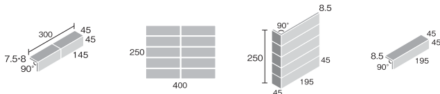
形状図
